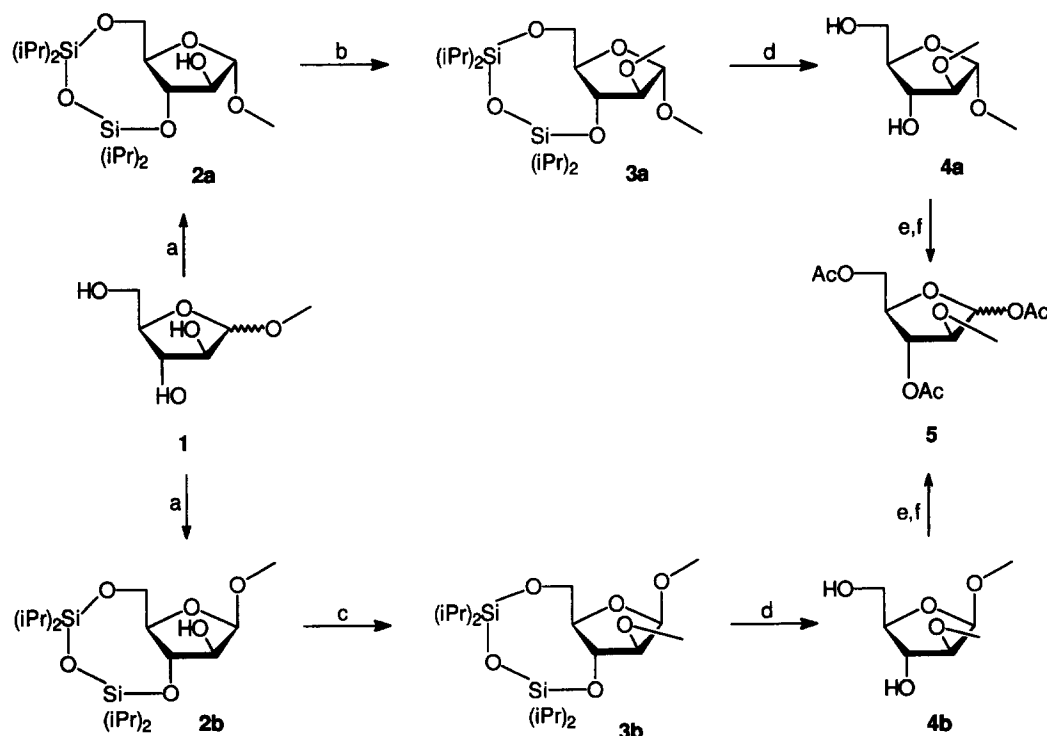
Scheme 1. (a) TIPDSCl 2 , anhydrous pyridine, anhydrous ClCH 2 CH 2 Cl; (b) BDDDP, CH 3 I, anhydrous CH 3 CN; (c) NaH, CH 3 I, anhydrous DMF; (d) Bu 4 NF in THF; (e) Ac 2 O, anhydrous pyridine; (f) glacial AcOH, Ac 2 O, conc H 2 SO 4 .
